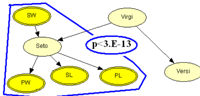
FIG. 5 – Réseau bayésien des données Iris (HuginLiteR8, algorithme Rebane-Pearl Polytrees). En noir les flèches correspondant à p < 0.05 , Dans la zone bleue celles qui restent en imposant p < 3.10^{-13} .
