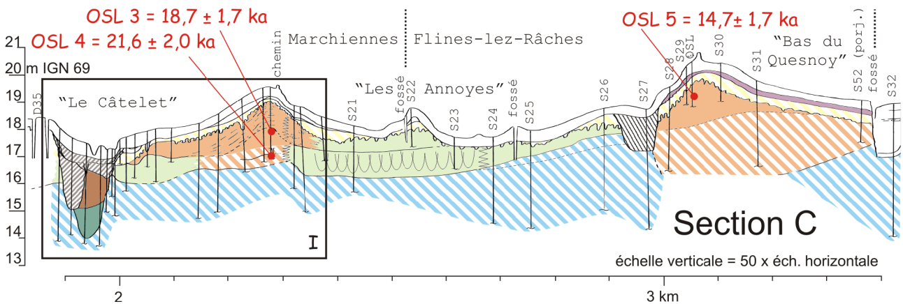
Illustration 29 - Transect gazoduc, section C cadre I, transect du câtelet, illustration suivante
