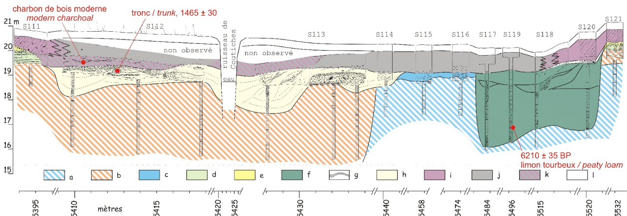
Illustration 27 - Transect du franchissement du ruisseau de Coutiches
