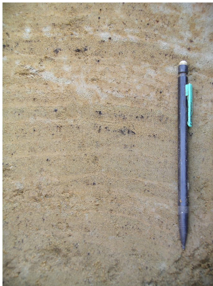
Illustration 33 - Détail du faciès éolien de la dune du Câtelet (unité 7)
