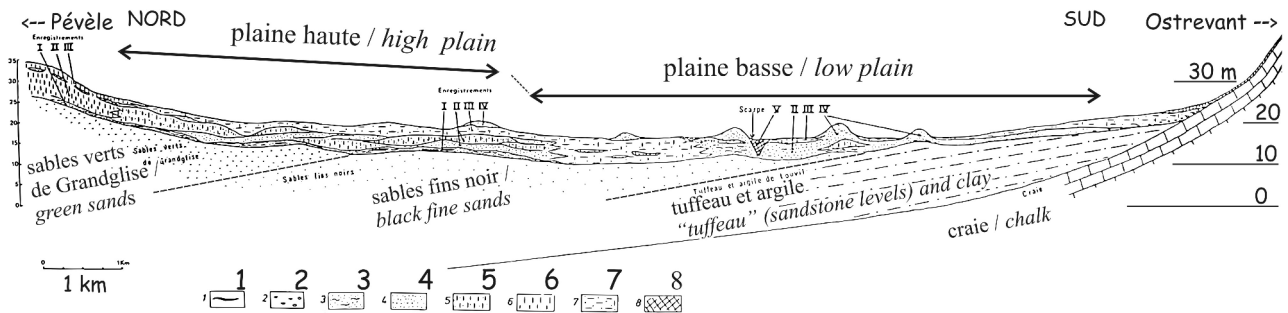
Illustration 3 - Coupe schématique des formations superficielles dans la partie est de la plaine
