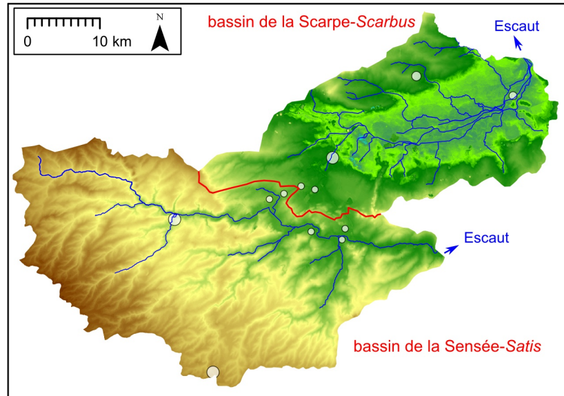
Illustration 6 - Les bassins Scarpe (Scarbus) – Sensée (Satis) avant la capture
