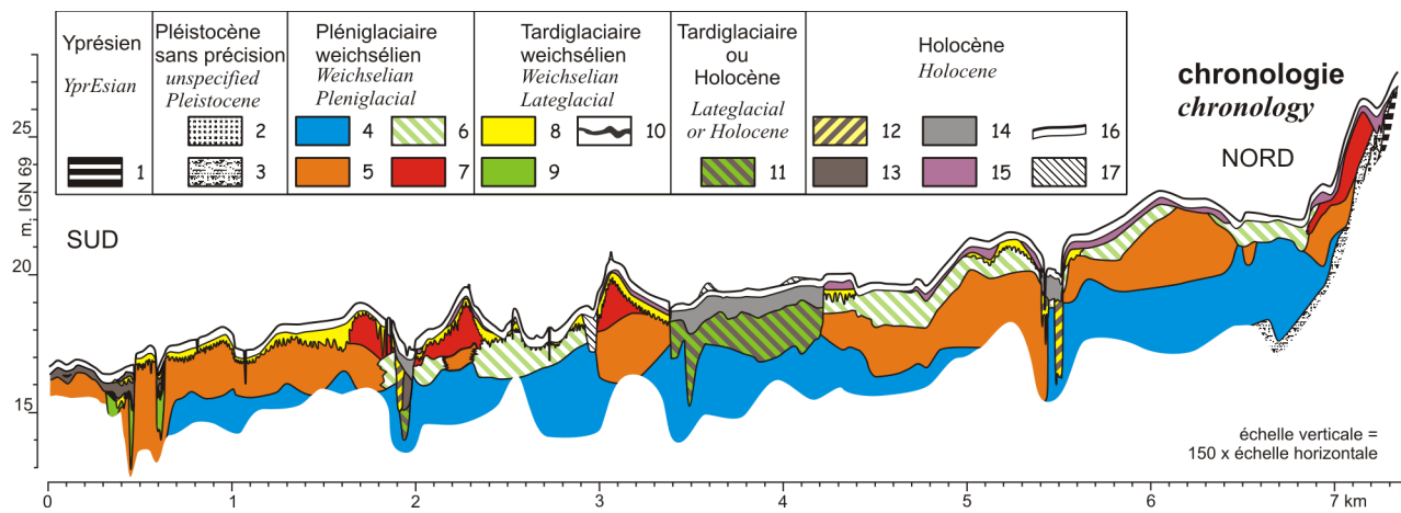
Illustration 12 - Interprétation chronostratigraphique
