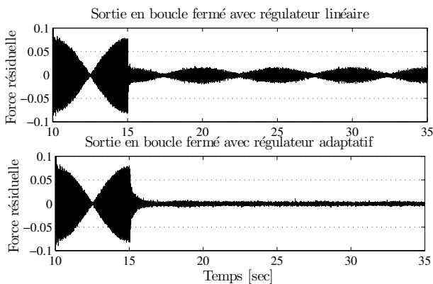
FIGURE 8 – La force résiduelle avec le régulateur linéaire robuste (courbe du haut) et avec le régulateur adaptatif (courbe du bas). La boucle est fermée à t=15 sec.
