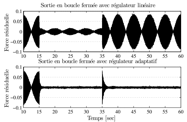
FIGURE 10 – La force résiduelle suite à un saut de fréquences de 5 Hz en boucle fermée avec le régulateur robuste (courbe du haut) et avec le régulateur adaptatif (courbe du bas). La boucle est fermée à t=15 sec.
