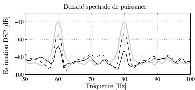
FIGURE 9 – Densité spectrale de puissance pour la boucle ouverte (gris), avec le régulateur linéaire robuste (pointillé) et avec le régulateur adaptatif (trait plein noir) dans la zone 50 à 100 Hz).
