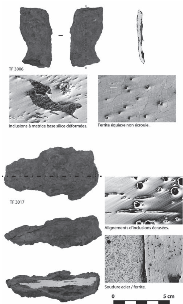
Figure 10 : Les chutes métalliques (chutes de fer plat) : caractéristiques macroscopiques et structurales. Figure 10: Metallic waste (flattened pieces of iron): macroscopic and structural characteristics.
