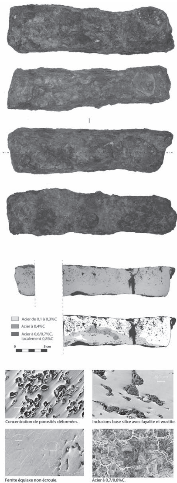
Figure 9 : Le demi-produit TF4 : caractéristiques macroscopiques et structurales. Figure 9: The semi-product TF4: macroscopic and structural characteristics.
