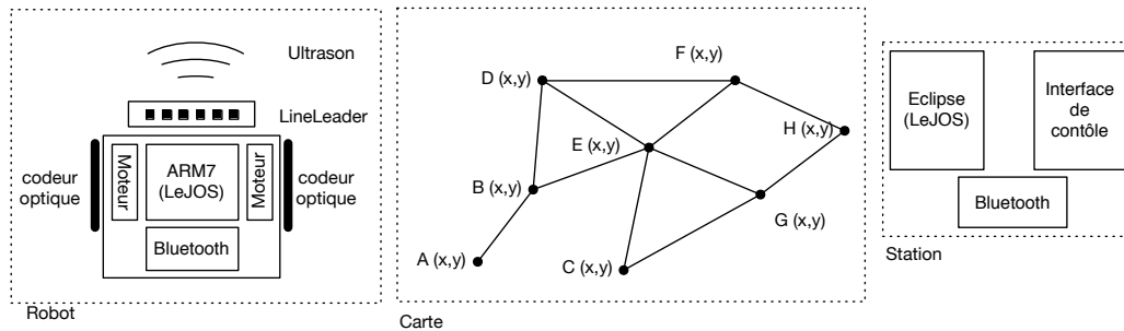
FIGURE 3 – Schéma de principe du robot, de la carte et de la station
