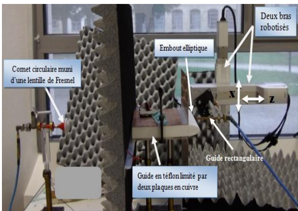
Figure 2. Dispositif expérimental
