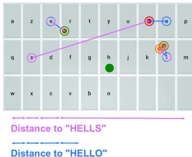
Fig. 3. : Illustration visuelle du fonctionnement du clavier DUCK (la version évaluée par les utilisateurs déficients visuels était invisible à l'écran). Une fois que l'utilisateur a tapé 5 lettres « au jugé », l'algorithme calcule des scores de proximité avec des mots du dictionnaire. Ici, il apparaît que la saisie est plus proche du mot 'HELLO' que du mot 'HELLS'. Le mot 'HELLO' sera proposé en premier. L'utilisateur pourra le valider ou passer au second choix avec une interaction gestuelle simple.
