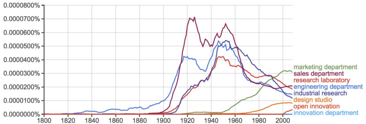
Figure 2 : Evolution de la fréquence relative de quelques termes classiques dans le corpus Google Books au cours du temps (outil Google Ngram) (langue anglaise)
