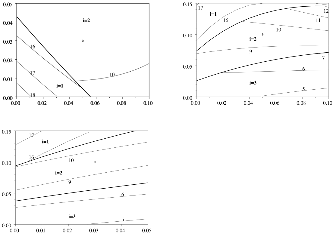
图2.当死亡率 \alpha 变化，贴现率 \beta 和每次收获的固定成本时的最佳周期长度和直径 c' 。左上方：图 (\alpha, \beta) 。右上：图 (\alpha, c'/NPV_\infty) 。底部：图 (\beta, c'/NPV_\infty) 。粗线将 i = 1 （均匀管理是最佳）的区域与 i = 2 和 i = 3 （均匀管理是最佳）的区域分开。其他线是用于最佳切割周期长度的水平线。在每种情况下，一个点都会调用图1中的参数值。
