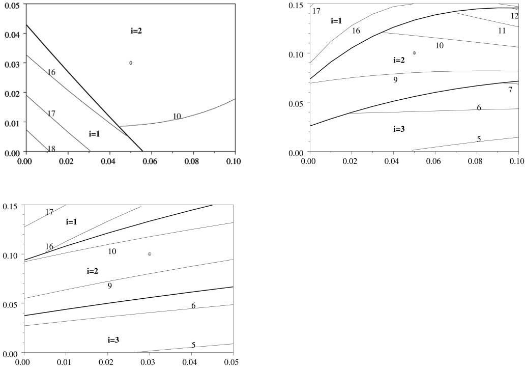
Figura 2. Comprimento e diâmetro ótimos do ciclo quando a mortalidade \alpha varia, a taxa de desconto \beta e o custo fixo por colheita c' . Superior esquerdo: diagrama (\alpha, \beta) . Superior direito: diagrama (\alpha, c'/NPV_\infty) . Parte inferior: diagrama (\beta, c'/NPV_\infty) . As linhas em negrito separam as áreas em que i = 1 (o gerenciamento uniforme é ideal) das áreas em que i = 2 e i = 3 (o gerenciamento desigual é ideal). As outras linhas são as linhas de nível para a duração ideal do ciclo de corte. Em cada caso, um ponto recupera os valores dos parâmetros na Figura 1.
