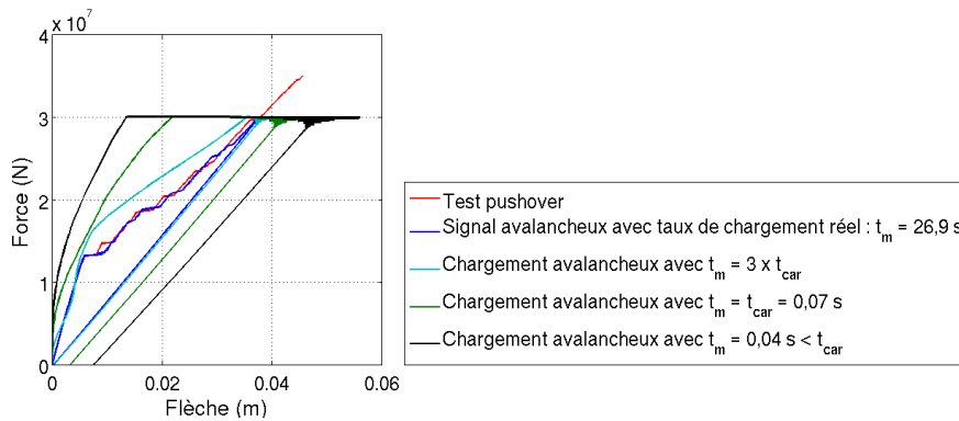
Figure 10 – Réponses de la structure à différentes sollicitations avalancheuses
