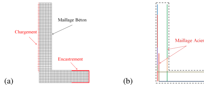
Figure 3 – Maillage modèle réduit : (a) béton et (b) acier et conditions aux limites (a)
