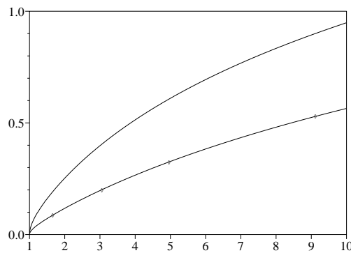
FIGURE 2 – La vitesse sans dimension \sqrt{X^*} = v^*/\sqrt{b_2 d} en fonction de \alpha_2/\alpha_1 pour différentes valeurs de y = b_2/b'_2 , à savoir y = 0,04 (en bas) et y = 0,1 (en haut). Les points correspondent à des simulations numériques du système non linéaire d'équations aux dérivées partielles.
