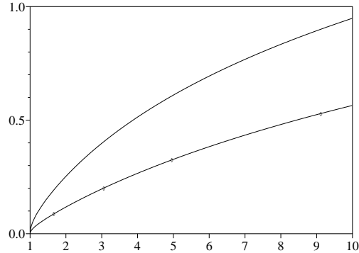
FIGURE 2 – La vitesse sans dimension \sqrt{X^*} = v^*/\sqrt{b'_2 d} en fonction de \alpha_2/\alpha_1 pour différentes valeurs de y = b_2/b'_2 , à savoir y = 0,04 (en bas) et y = 0,1 (en haut). Les points correspondent à des simulations numériques du système non linéaire d'équations aux dérivées partielles.
