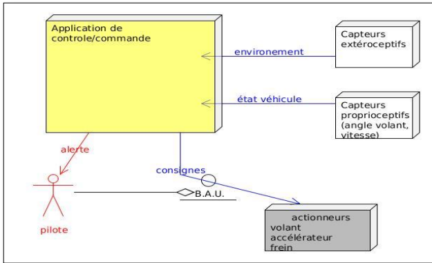
Figure1: Schéma de déploiement UML simplifié
