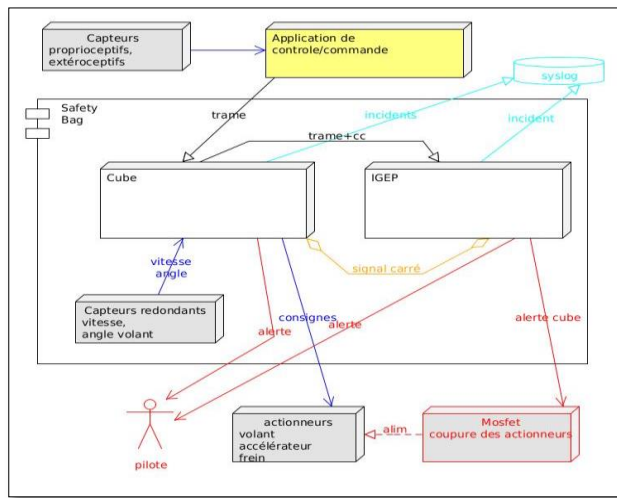
Figure5: Schéma de déploiement UML simplifié
