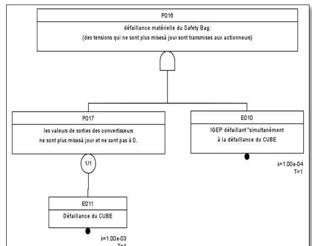
Figure6: Arbre de défaillances
