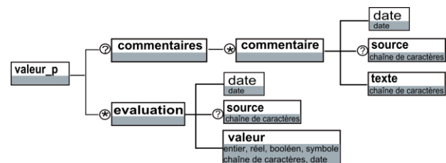
Figure 4 : Représentation graphique de valeur_p dans PMDL e .
