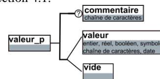
Figure 3 : Représentation graphique de valeur_p dans PMDL.
