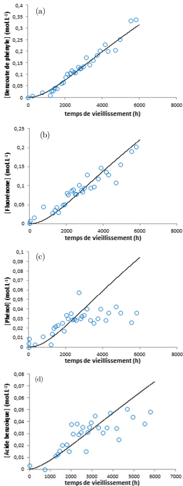
Fig. 12. Simulation de l'évolution des concentrations en benzoate de phényle (a), fluorénone (b), phénols (c) et acide benzoïque (d) au cours du vieillissement thermique du PEEK dans l'air à 523 \text{ K} .
