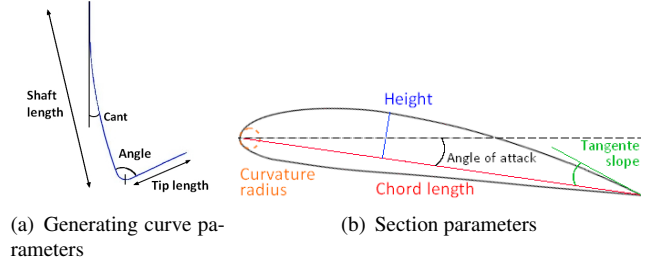
Figure 3: Foil parameters
