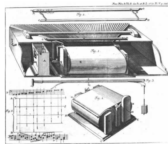
Figure 3 : Johann Georg Sulzer, « Description d'un instrument fait pour noter les pièces de musique, à mesure qu'on les exécute sur les clavecins » , Nouveaux mémoires de l'Académie Royale des Sciences et Belles-Lettres , Berlin, 1771.
