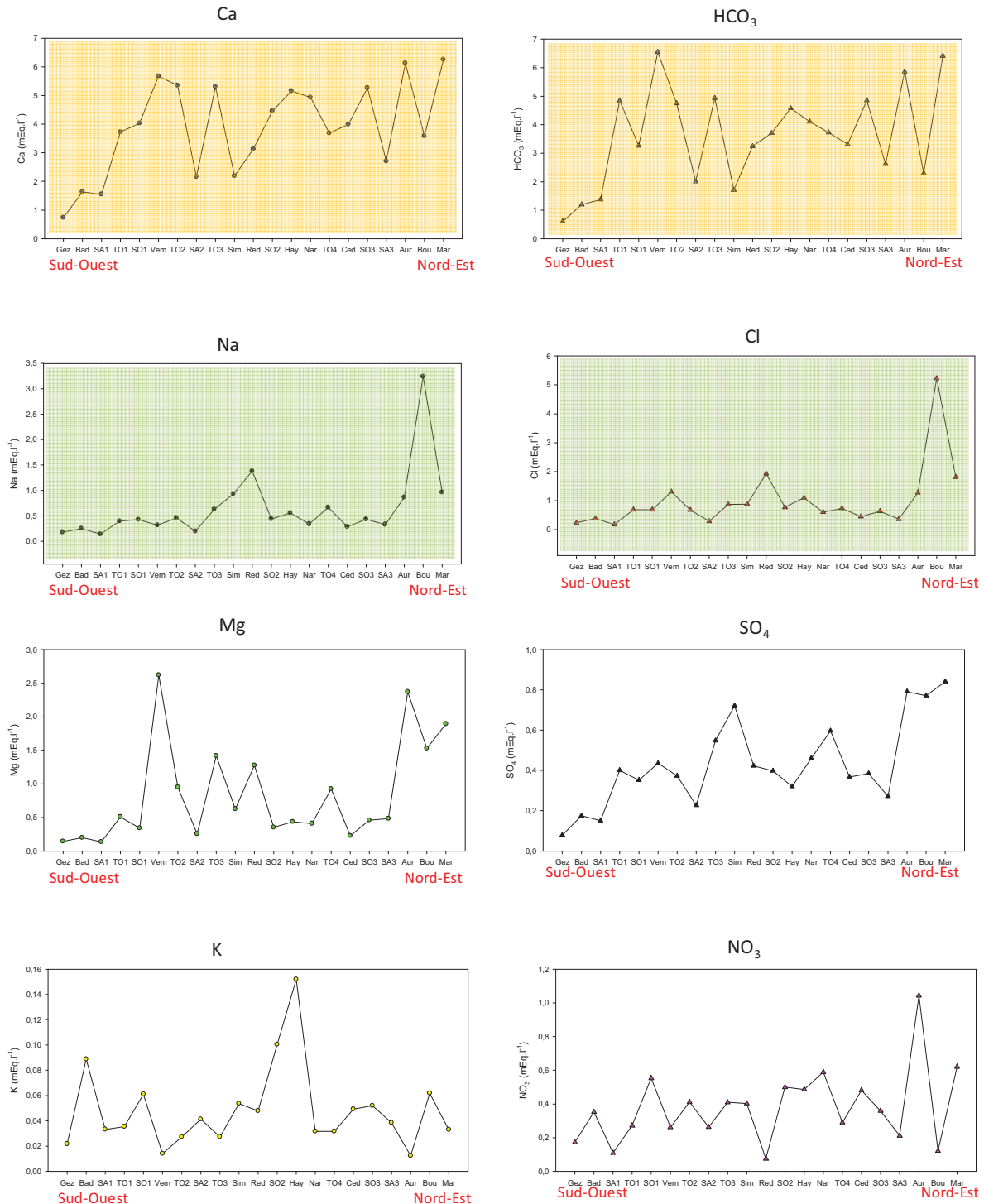
Figure 6 : Variabilité spatiale des cations et anions majeurs dans les cours d'eau de la Gascogne
