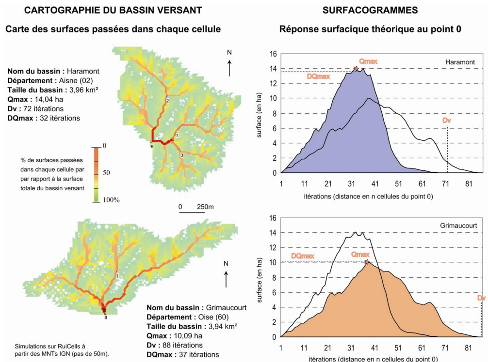
Figure 7 : Importance de l'organisation spatiale des surfaces et des réseaux au sein des bassins versants : Deux surfacoigrammes différents pour des bassins de taille similaire
