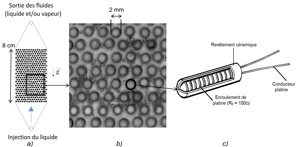
Figure 1 : a) Schéma de la section ; b) Exemple de visualisation ; c) Schéma d'un élément chauffant.
