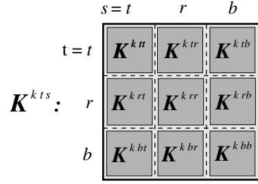
Fig. 4. Basic scheme of layer arrays \mathbf{K}_{ij}^{kts} ( i, j = u, e ).
