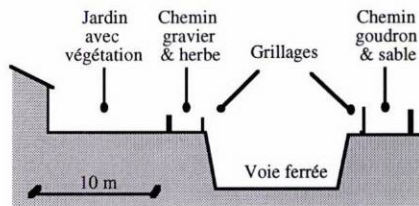
Coupe sur parcours
