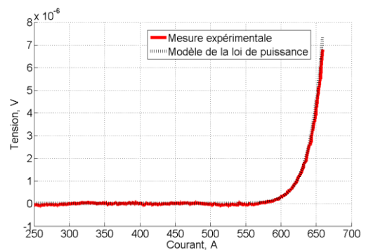
Fig.5 Transition d'un échantillon TRBCO de son état supraconducteur à son état dissipatif sous 8 T avec angle d'incidence de 10°, résultat expérimental et modèle appliqué sur la mesure.
