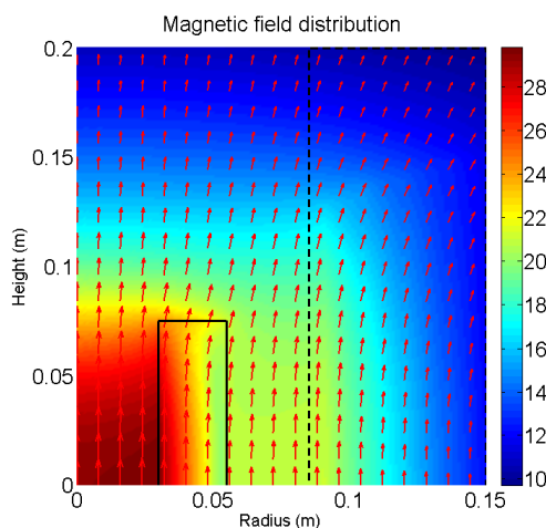
Fig.2 Distribution du champ magnétique dans l'assemblage insert SHTC 10 T dans l'aimant extérieur résistif 20 T, graphique issu du logiciel FLUX ® .
