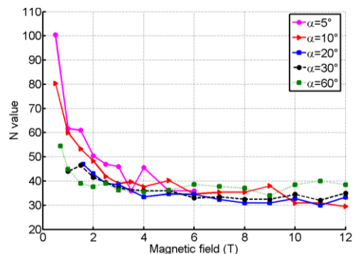
Fig.6 Valeur du facteur de puissance en fonction du champ magnétique pour différents angles d'incidence.
