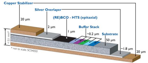
Fig.1 Exemple d'une coupe d'un ruban supraconducteur, issu des données SuperPower® [10].
