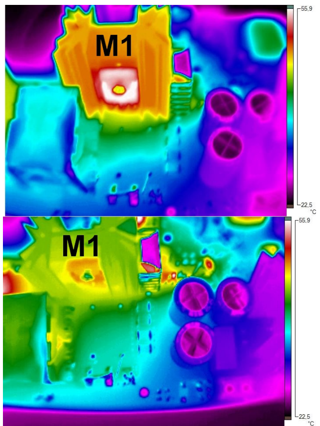
Fig.12 Imagerie thermique du transistor M_1 , convertisseur à 120V-30W en temps mort fixe (haut) et en temps mort variable (bas).
