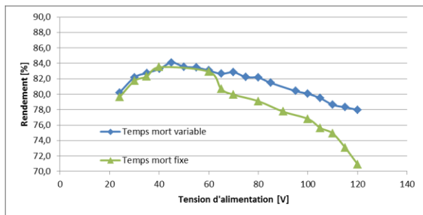
Fig.9 Rendement du convertisseur 30 W en fonction de la commande.
