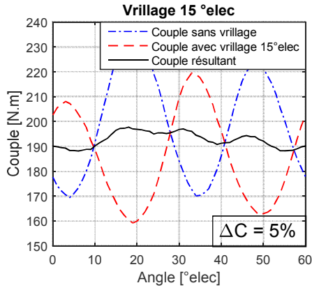
Fig.9. Ondulation de couple sans et avec vrillage du rotor de 15°elec
