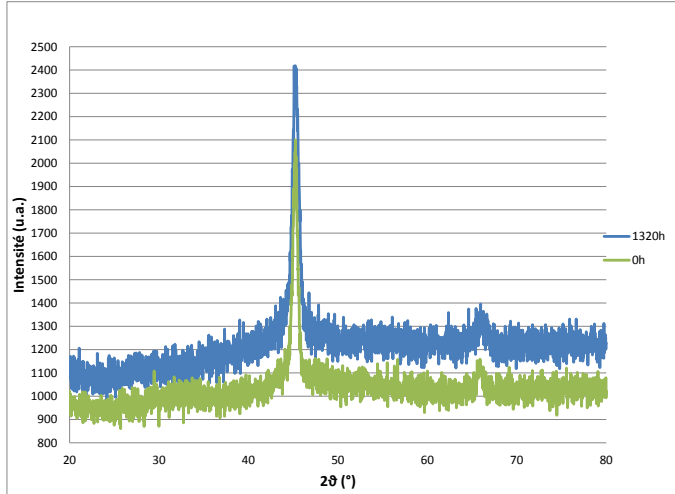
Fig. 9 Diffractogrammes DRX du \mu 500000 non vieilli et vieilli à 240°C pendant 1320 heures
