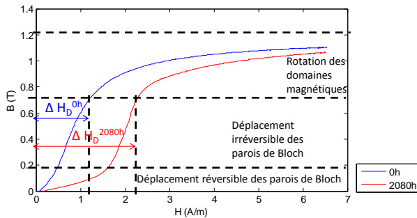
Fig. 12 Représentation des régions de déplacement des parois de Bloch et de rotation des domaines magnétiques sur les courbes de première aimantation avant et après vieillissement de 2080h à 240^\circ\text{C} .
