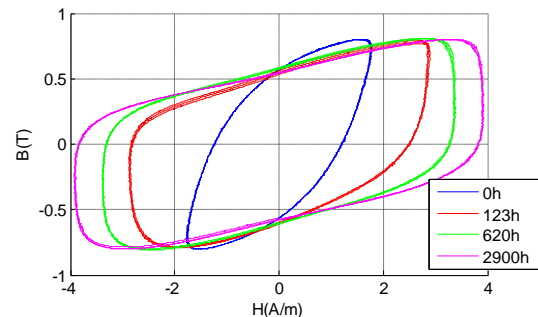
Fig. 6 Cycles d'hystérésis à 0,8 T/1 kHz pour plusieurs durées de vieillissement à la température de 240^\circ C .
