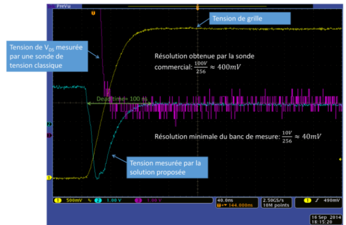
Figure 2 : Illustration de l'amélioration de la résolution obtenue avec le banc étudié (courbe bleue) comparée à la résolution atteinte avec une sonde commerciale (courbe violette) immédiatement après la mise en conduction du composant (100 ns).
