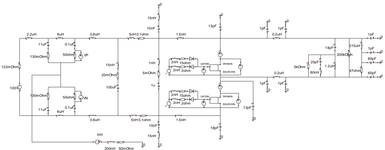
Fig. 9 Modèle complet
