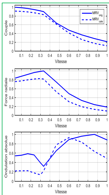
Fig. 7 Comparaison en fonctionnement, MRV orig vs. MRV cale
