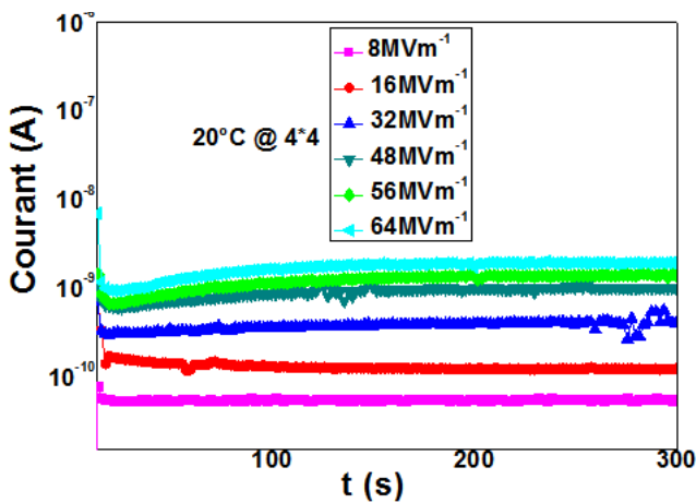
Fig.8 Caractéristiques I-t sous l'effet d'une précontrainte symétrique pour différents champs électriques appliqués à l'ambiante.
