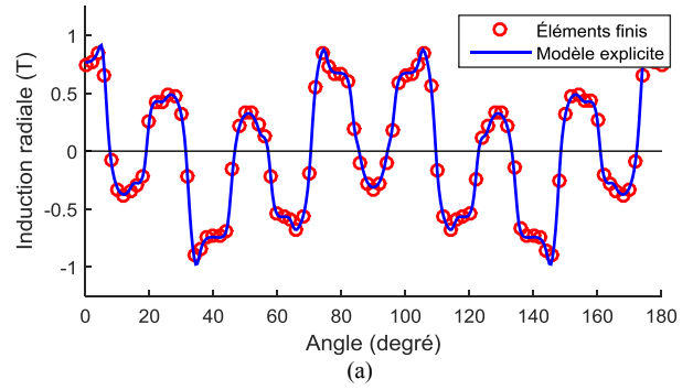
Fig.5 Composantes radiale (a) et tangentielle (b) de l'onde d'induction au rayon moyen de l'entrefer intérieur avec p_h = 2 , p_l = 7 , Q = 9 .
