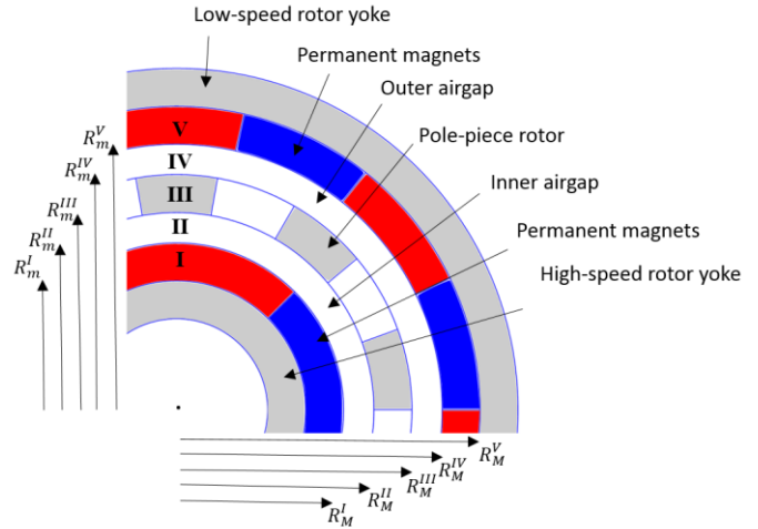
Fig.3 Numérotation des cinq régions du multiplicateur prises en compte dans le modèle explicite (exemple avec : p_h = 2, p_l = 7, Q = 9 ).
