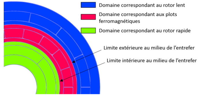
Fig.7 Définition des différents domaines solidaire pour l'étude par éléments finis magnétodynamique avec les limites intérieure et extérieure entre ces trois domaines pour p_h = 2, p_l = 7, Q = 9 .
