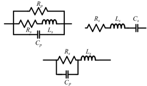
Fig. 7: Modèle haute fréquence d'une bobine, d'un condensateur et d'une résistance (de gauche à droite)
