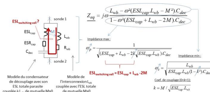
Fig. 11 Modèle circuit équivalent à constantes localisées et couplées de l'impédance d'une maille de commutation. Identification basse-fréquence de résonance et du coefficient de couplage (les valeurs basse-fréquence et haute-fréquence de l'inductance équivalente "vues des bornes" peuvent aussi aisément être déduites). WB : fils bonding.
