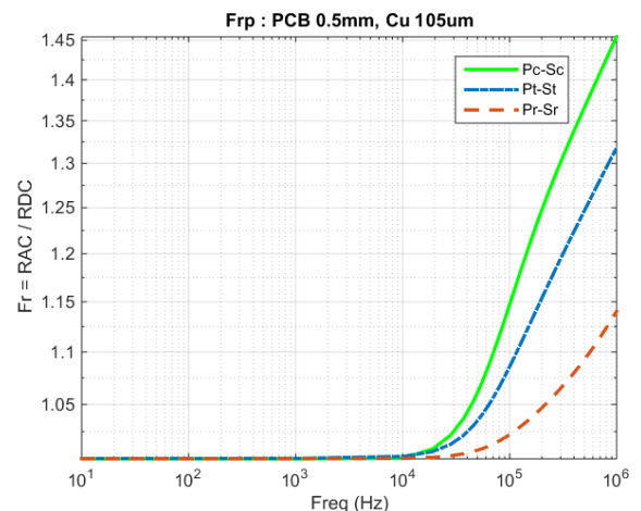
Fig.3 Comparaison des facteurs résistifs primaires ( F_{rp} ) de trois combinaisons (Cu 105µm et PCB 0.5mm).
