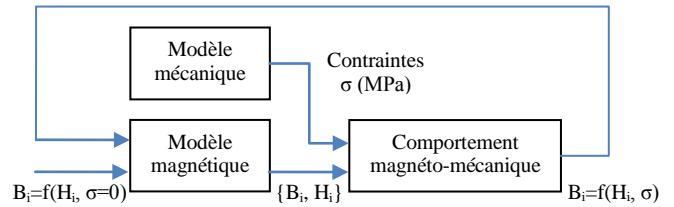
Fig. 6 Schéma du couplage magnéto-mécanique.
