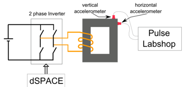
Figure 5: Banc expérimental et mesures vibratoires.
