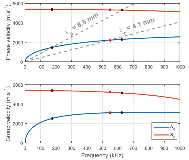
FIGURE 3 – Courbes de dispersion des modes A_0 et S_0 . Points noirs : vitesses relative à une amplification de mode; points rouges : vitesses relative à une atténuation de mode.
