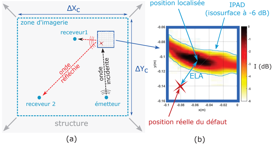
FIGURE 1 – Illustration du processus d'imagerie par réflexion d'ondes guidées (a) ; exemple typique d'une image générée (b).
