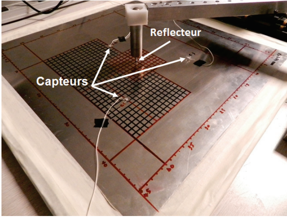
FIGURE 2 – Système expérimental.
