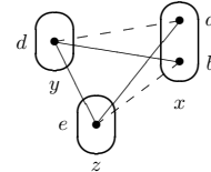
FIGURE 1 – Un triangle cassé sur deux valeurs a, b d'une variable x donnée.
