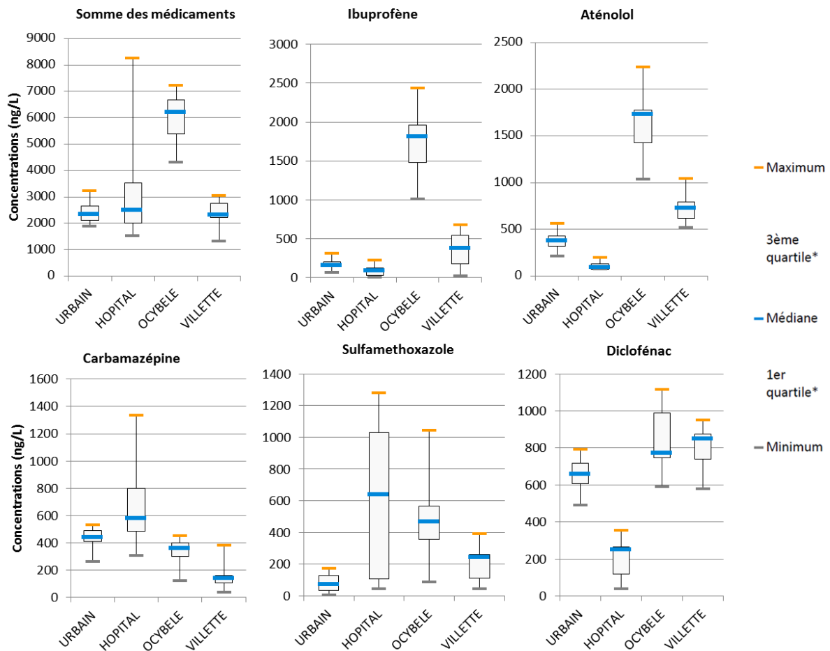
Figure 3. Concentrations en ng/L des rejets de stations d'épuration (STEP) (Janvier 2013 à Janvier 2015; 9 campagnes)
