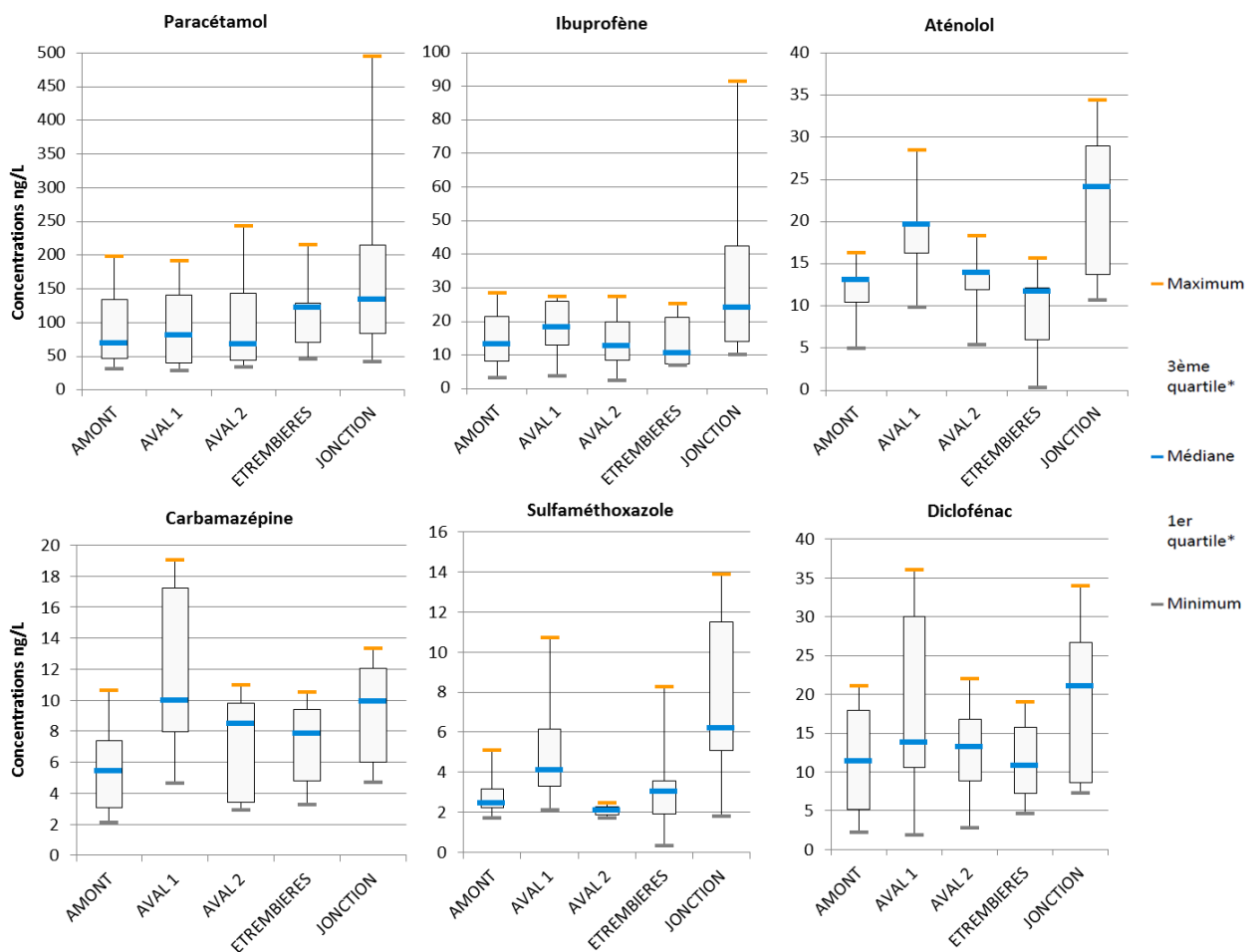
Figure 4. Concentrations en ng/L dans l'Arve (Janvier 2013 à Janvier 2015; 9 campagnes)
