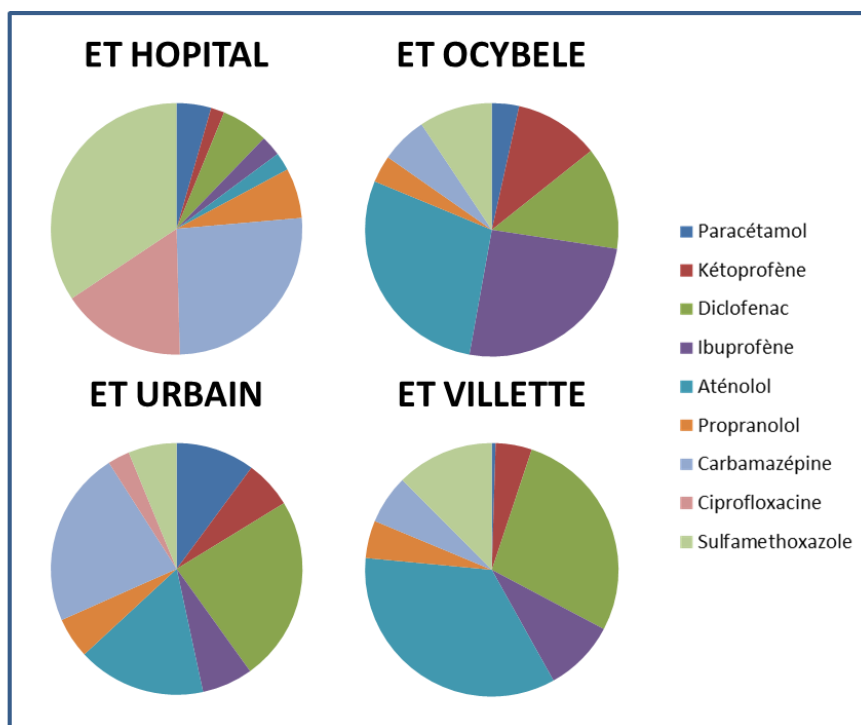
Figure 2. Contribution de chaque composé à la somme des substances analysées dans les eaux en sorties des stations d'épuration étudiées – Observatoire SIPIBEL-IRMISE (Janvier 2013 à Janvier 2015 ; 9 campagnes)
