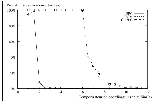
Figure 14. Pb_{ISW} vs temporisateur du coordinateur.
