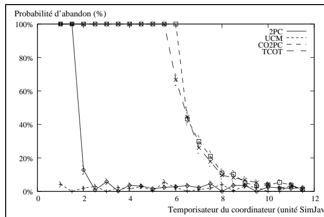
Figure 15. Pb_{ab} vs temporisateur du coordinateur.
