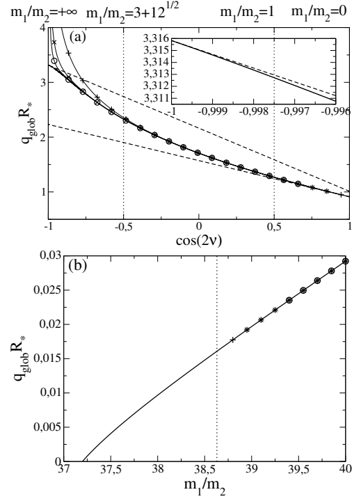
Figure 3. Valeur de q_{\text{glob}} R_* donnant l'échelle d'énergie globale E_{\text{glob}} = \hbar^2 q_{\text{glob}}^2 / 2m_r [ou de manière équivalente le paramètre à trois corps R_t selon les eqs. (13,19)] pour deux bosons identiques de l'espèce 1 et une particule d'espèce différente 2 interagissant avec une longueur de diffusion infinie dans l'onde s sur une résonance de Feshbach étroite, en fonction du rapport de masse m_1/m_2 ou de l'angle de masse \nu = \arcsin \frac{m_1}{m_1+m_2} , dans le secteur de moment cinétique \ell = 0 pour (a) et \ell = 2 pour (b). Trait plein épais : valeur exacte éq. (31), à la fois pour le cas préefimovien limité à s_\ell \in ]0, 1/2] [dans (b) à gauche de la ligne pointillée verticale] et pour le cas efimovien s_\ell \in i\mathbb{R}^+ [partout dans (a) et à droite de la ligne pointillée verticale dans (b)]. Symboles reliés par des traits fins : dans le cas efimovien, à partir des estimations E_{\text{glob}} \simeq -\epsilon_q \exp[2\pi(q+1)/|s_\ell|] (exactes pour q \rightarrow +\infty ou |s_\ell| \rightarrow 0 ), où \epsilon_q est l'énergie du gème état trimère, q \in \mathbb{N} , obtenue numériquement à partir de l'éq. (23) quand c'est faisable ( q = 0 : plus, q = 1 : croix, q = 2 : cercles); quand m_1/m_2 \rightarrow +\infty la partie basse du spectre devient hydrogénoïde [46] (plutôt que géométrique) et (-2m_r \epsilon_q)^{1/2} R_* / \hbar \rightarrow +\infty , d'où les écarts à la courbe en trait plein noir épais. En (a) les droites obliques en tiretés sont les développements (36) et (37), ce dernier étant en réalité utile sur une plage très limitée, voir l'agrandissement dans l'encadré, et les lignes pointillées verticales repèrent les rapports de masse m_1/m_2 = 1 et 3 + \sqrt{12} où \cos 2\nu = \pm \frac{1}{2} . En (b), q_{\text{glob}} s'annule au rapport de masse tel que s_2 = 1/2 , mais il ne s'agit pas d'une véritable résonance à trois corps (voir le texte). La longueur de Feshbach R_* est liée à la portée effective à deux corps par r_e = -2R_* à l'unitarité.
