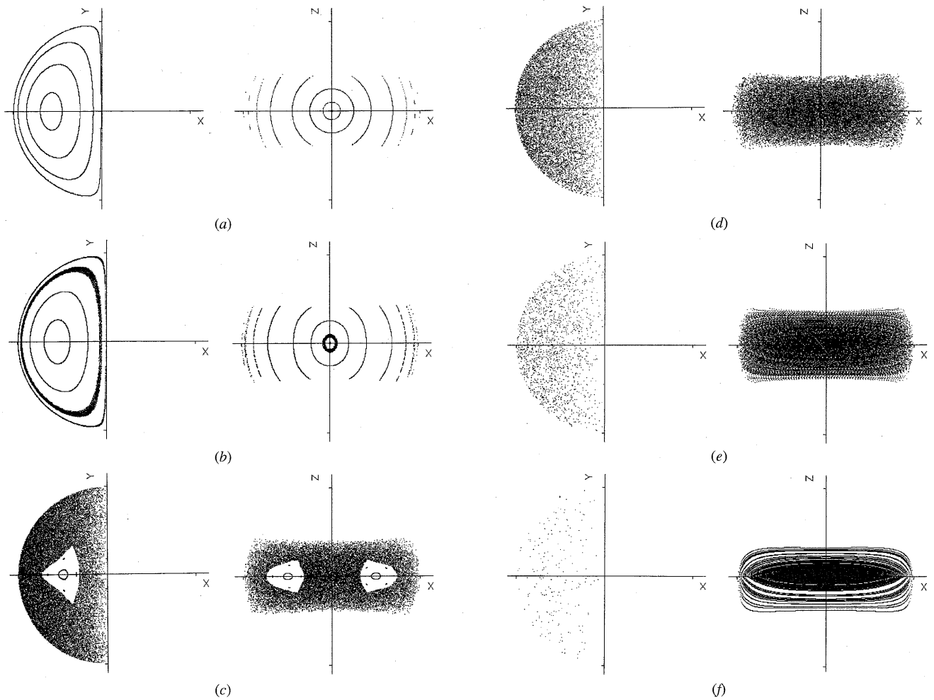
Sections de Poincaré z = 0 et y = 0 de l'écoulement \mathbf{u} = \mathbf{U} + \mathbf{V} , pour \alpha = : (a) 0,01, (b) 0,1, (c) 0,3, (d) 1, (e) 10, (f) 100.
