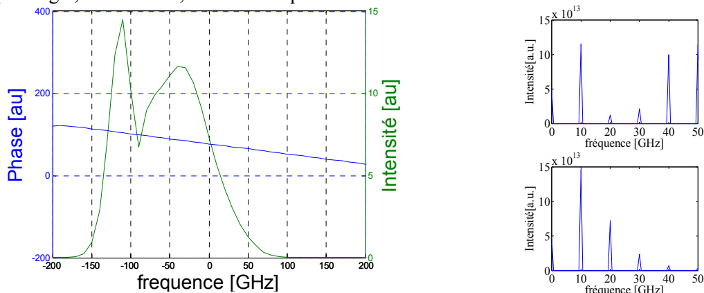
Fig. 4 : Intensité spectrale et distribution de phase du peigne de fréquences obtenu en simulation (gauche) et spectre RF obtenu après photodétection pour deux retards fibrés
