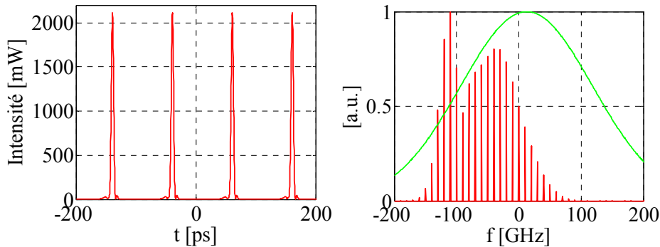
Fig. 3: Profil temporel (à gauche) et spectral (à droite) du train d'impulsions à 10 GHz
