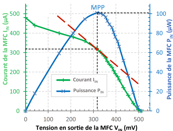
Fig. 3. Courbe de polarisation d'une MFC obtenue en faisant varier la tension V_{IN} par pas de 20mV/10min.
