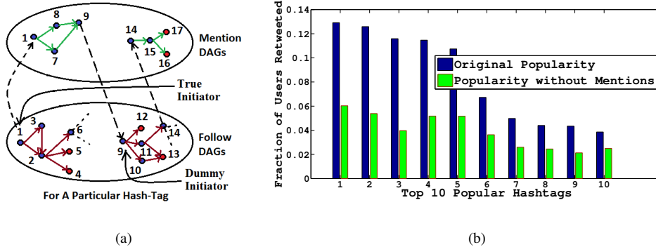
FIGURE 2. (gauche) Exemple de graphe multiplexe. (droite) Popularité des 10 hashtags les plus populaires de “Algeria” avec et sans mentions.
