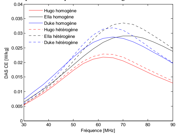
Figure 2 : DAS CE en HF et VHF pour différents fantômes exposés à une onde plane à 1 W/m 2
