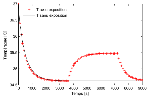
Figure 7 : Evolution de la température à 60 MHz au point de DAS 10g max pour Duke hétérogène – Exposition onde plane (61 V/m ; T_{ext} = 28\text{ °C} )
