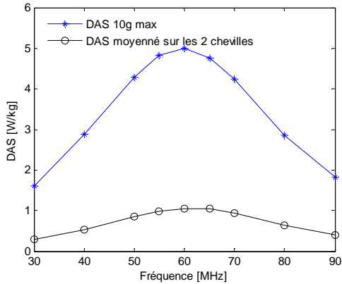
Figure 5 : DAS 10g max et DAS moyenné dans les chevilles pour Duke hétérogène - Exposition onde plane (61 V/m ; T_{ext} = 28\text{ °C} )
