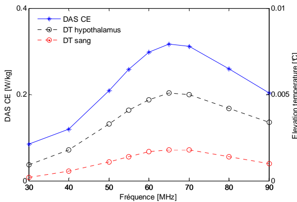
Figure 8 : DAS_{CE} et \Delta T dans le sang et l'hypothalamus pour Duke hétérogène - Exposition onde plane (61 V/m ; T_{ext} = 28\text{ °C} )
