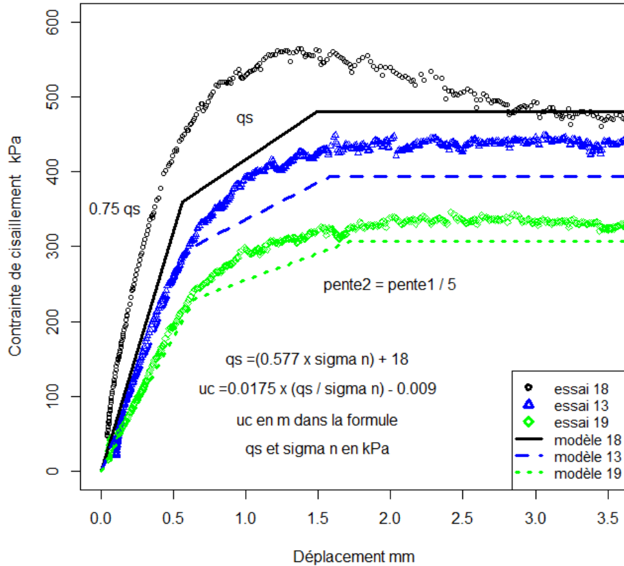
Figure 3. Contrainte moyenne de cisaillement en fonction du déplacement et modèle tri-linéaire pour les boulons cylindriques scellés à la résine Locket.
