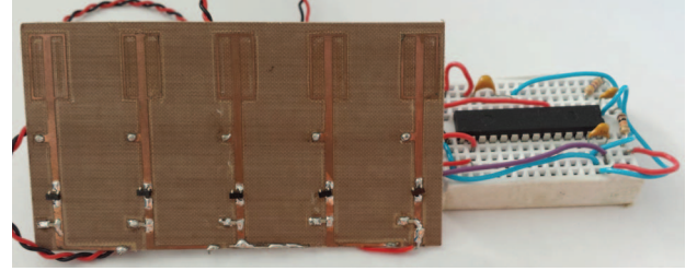
Fig. 3. Picture of the WuRx prototype.
